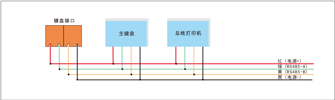
主机与主键盘、打印设备的连接示意图
