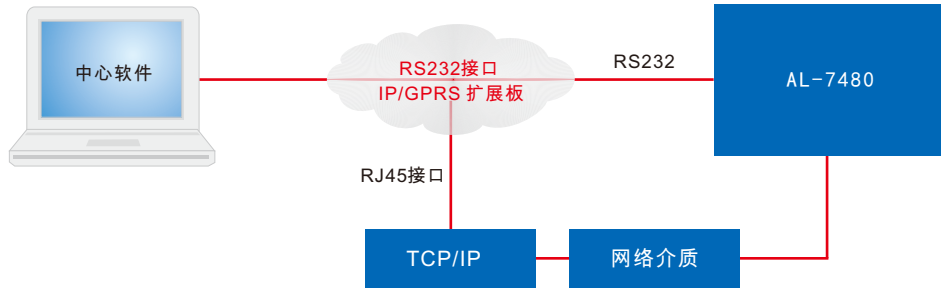
AL-74系列主机通过RS232或IP网络与中心连接示意图
